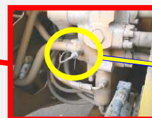
Rozvod hydraulického oleje do pístů zdvihu na lopatovém nakladači
